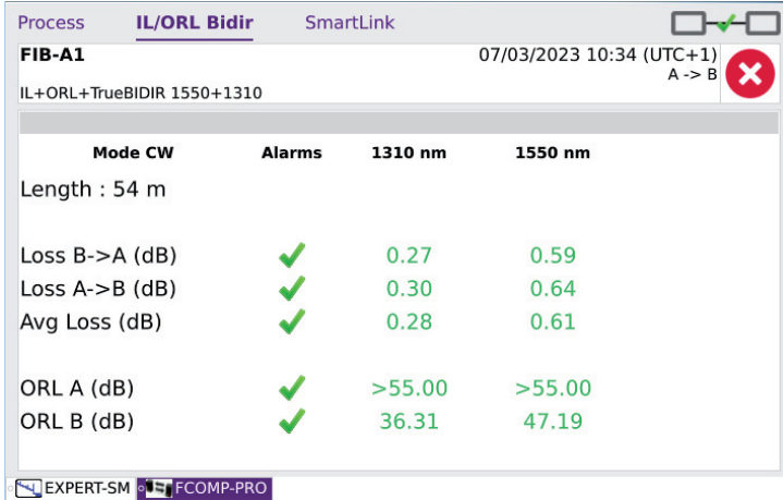
Results: Bidir IL/ORL
